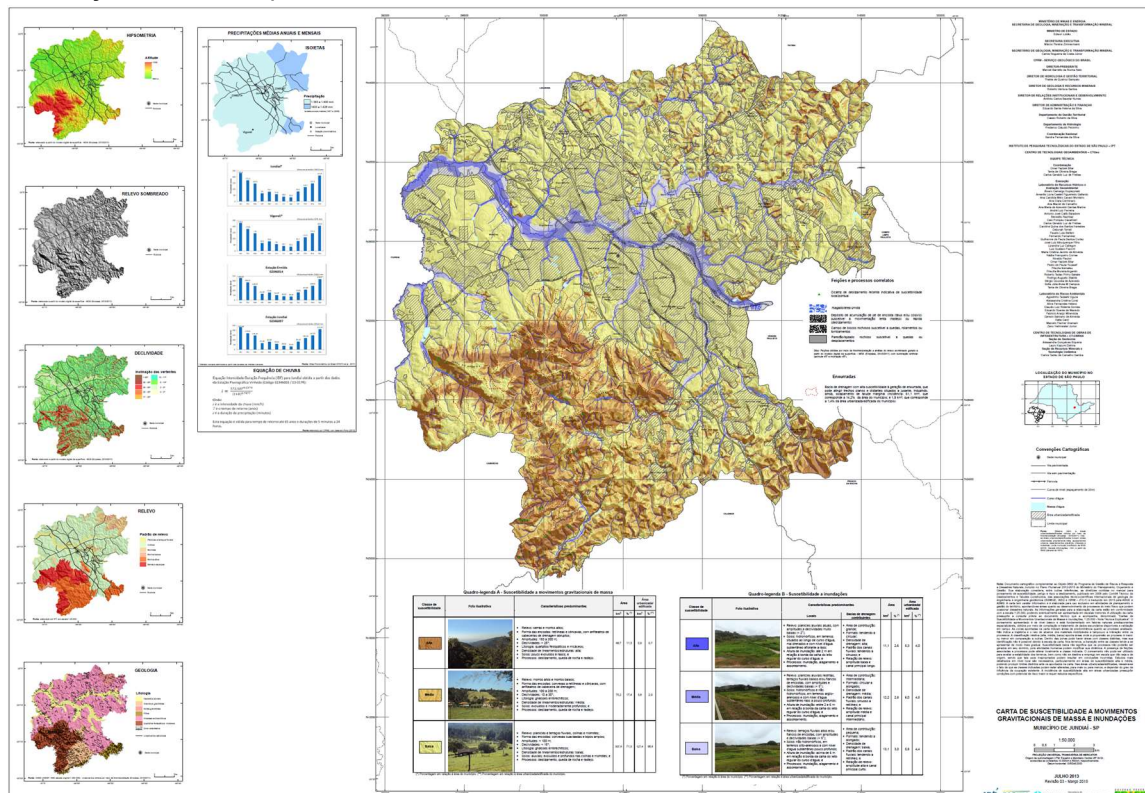
Figura 1- Ilustração da Carta de Suscetibilidade a Movimentos Gravitacionais de Massa e Inundações do Município de Jundiaí/SP.
