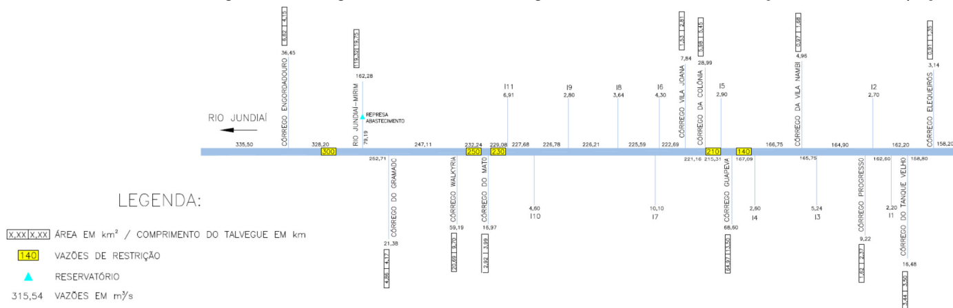
Figura 5.1 - Prognóstico da Macrodrenagem – TR – 10 anos – condição futura de ocupação
