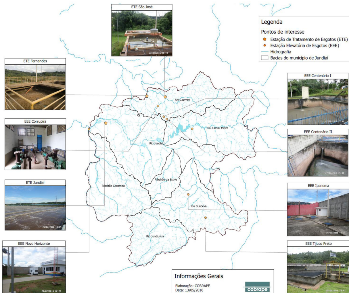
Figura 4.13 - Sistemas coletivos de esgotamento sanitário identificados em Jundiá
