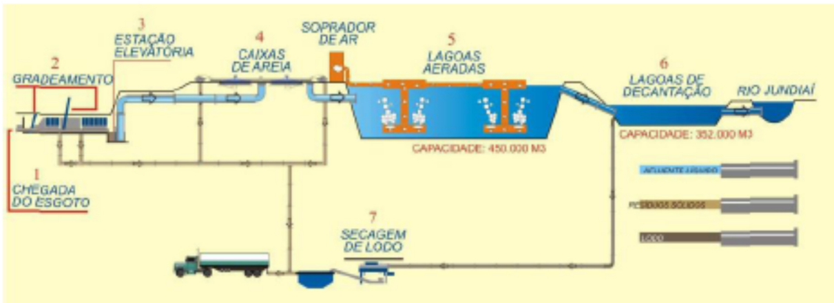
Figura 4.17 - Fluxograma da ETE Jundiáí
