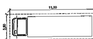
Dimensão mínima de vaga de carga e descarga (padrão)
