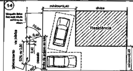
Situação permitida em residência unifamiliar.
