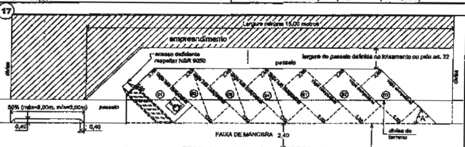
Situação não permitida para imóvel com testada inferior a 9,50m.
