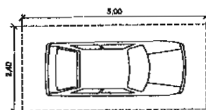
Dimensão mínima da vaga de auto
