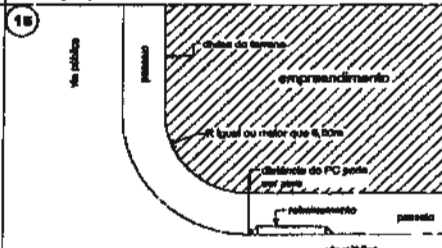
Rebatismo em esquina (raio maior ou igual a 6,00m)
