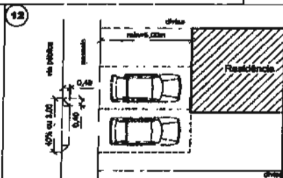
Situação permitida em residência unifamiliar.
