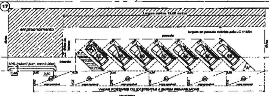
Vias Arteriais => "A" menor ou igual a 45° Vias Locais e Coletoras => "A" menor ou igual a 90°
