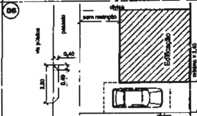
Imóvel com testada inferior ou igual a 8,00m.
