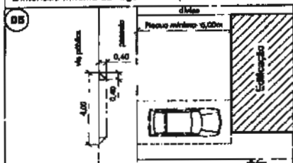
Imóvel com testada inferior a 8,00m, existentes na data de publicação da Lei Complementar nº 418/04.
